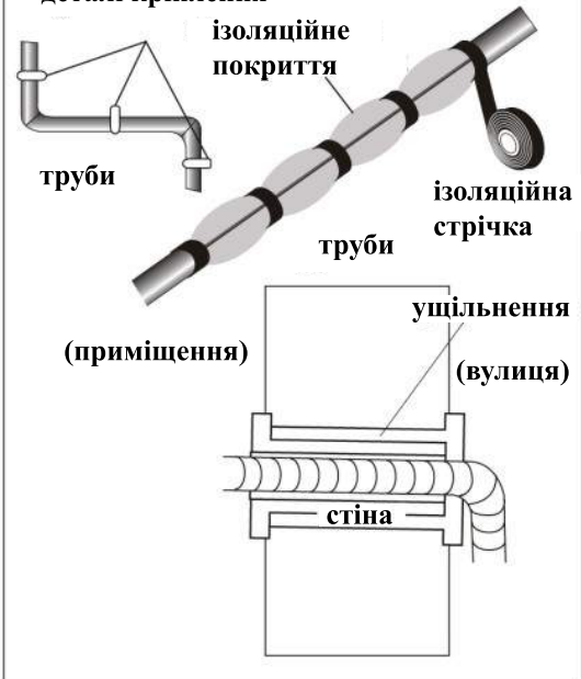
деталі кріплення
