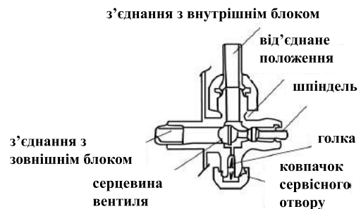
схема тристороннього вентиля
